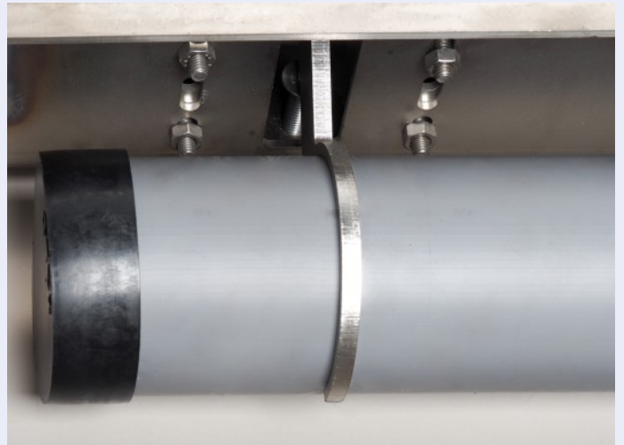
Details zum Schwimmer des MINI Klappschotts
